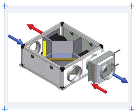
JR(H/V)(B)70
