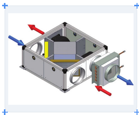
JR(H/V)(B)70
